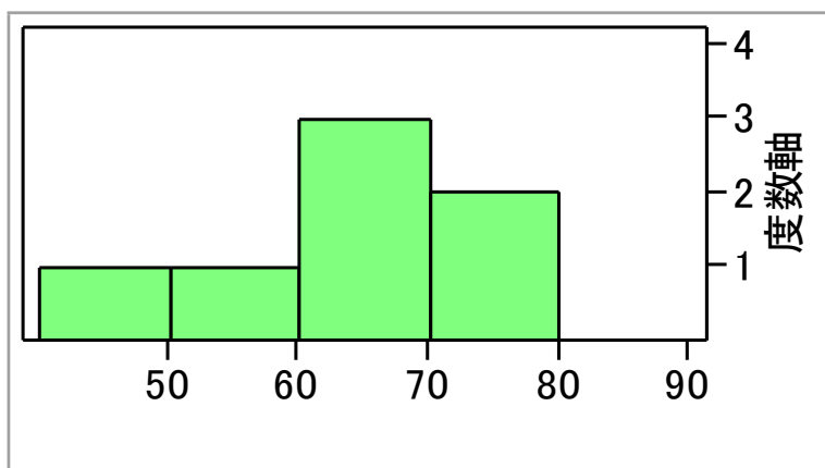
成績の分布
